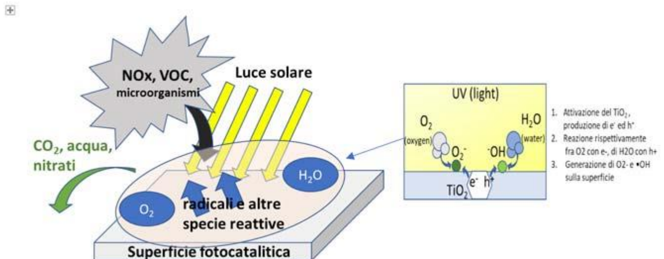
Figura 3 – Schema di meccanismo della fotocatalisi
